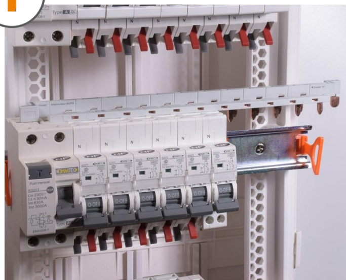
Exemple de montage avec disjoncteurs Auto
