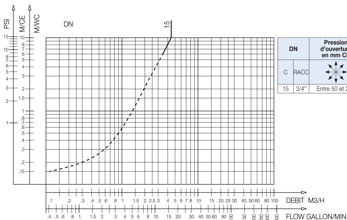
WF Compact Abaque des pertes de charge
