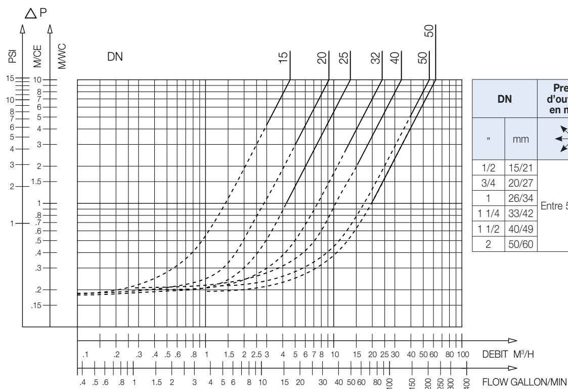
B.B. - Abaque des pertes de charge
