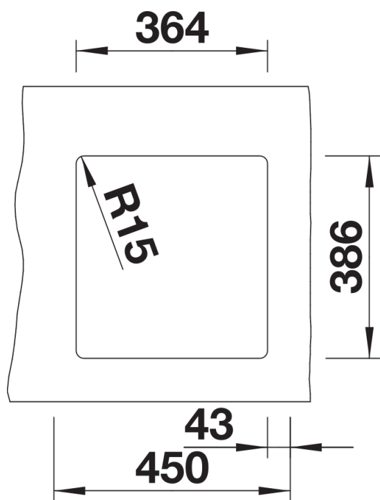
Découpe
