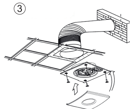
INSTALLATION DANS LE PLAFOND
