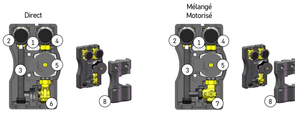
D&M (Direct + Mélangé Motorisé) avec COLLECTEUR
