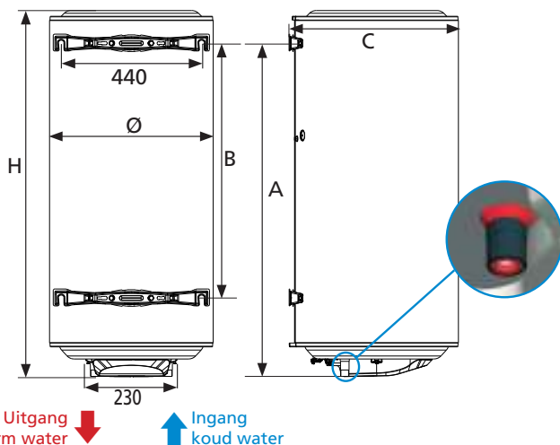
Schematische weergave
