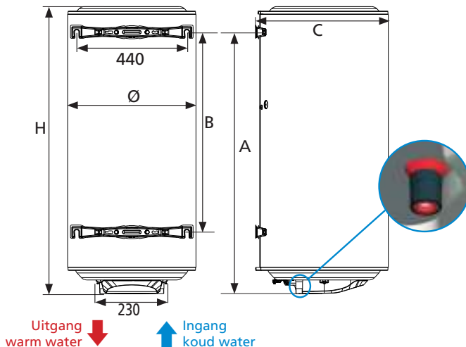
Schematische weergave
